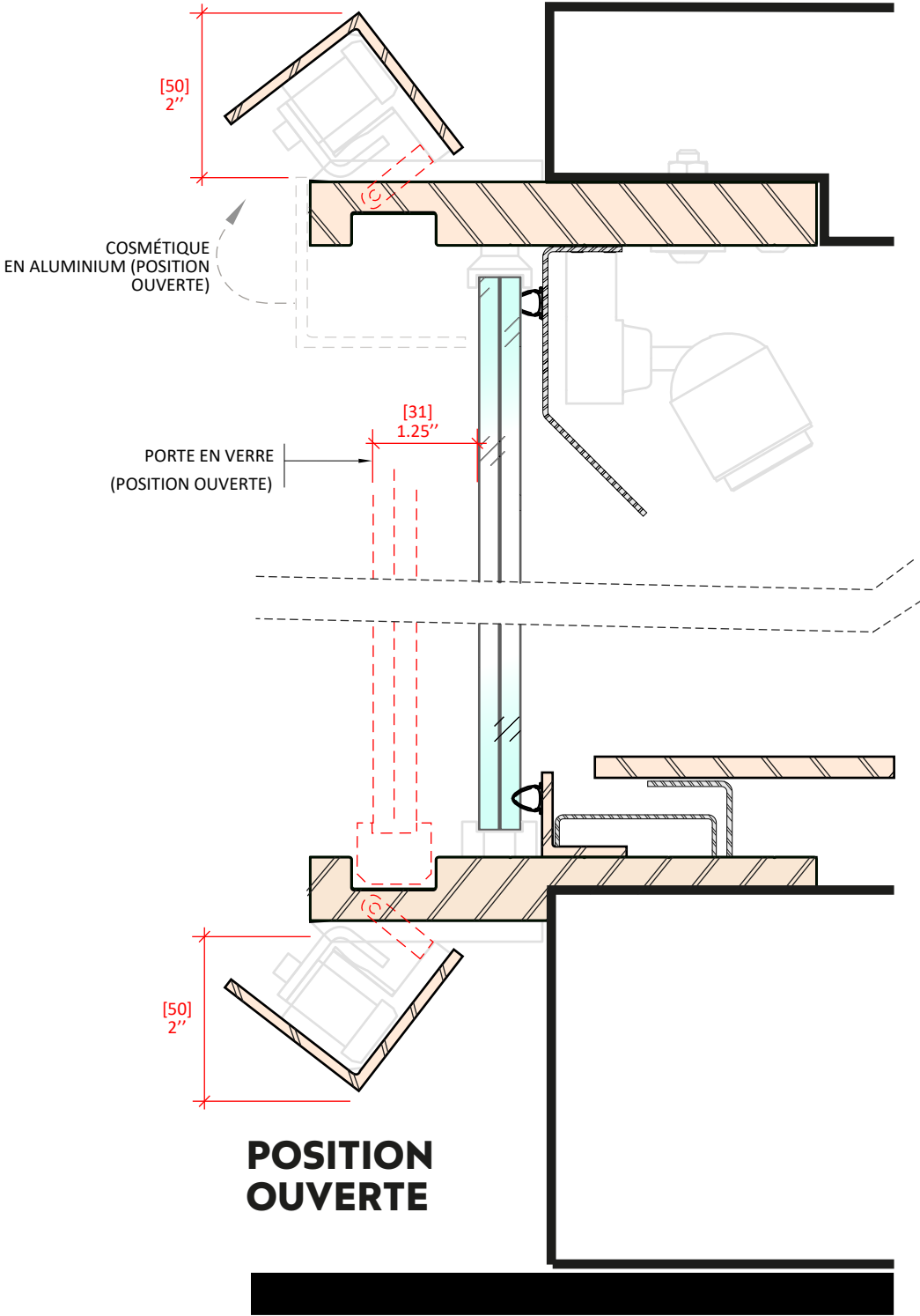
ÉCHELLE DE SECTION TYPIQUE 1:2
