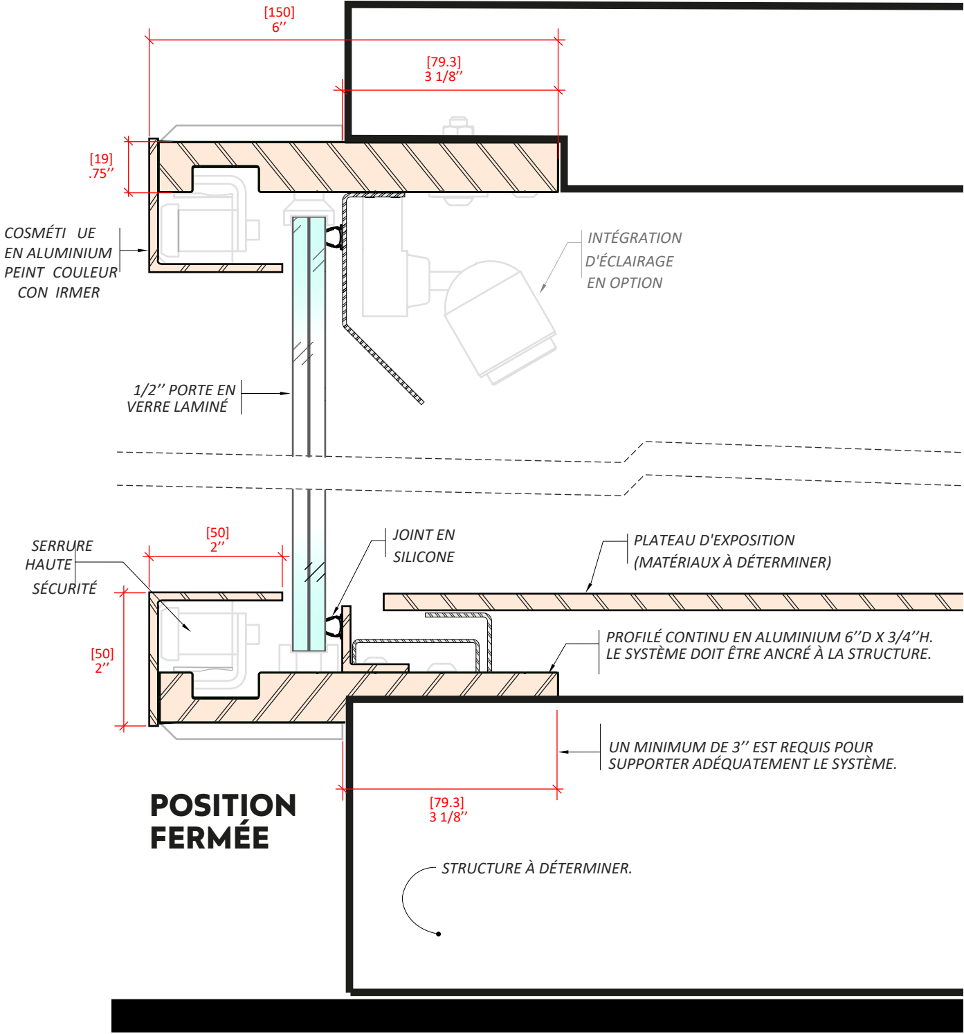
ÉCHELLE DE SECTION TYPIQUE 1:2
